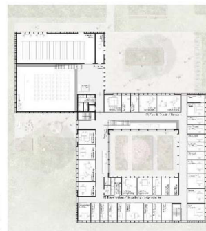
Grundriss Obergeschoss 35.1.2023
